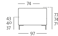
K-H-SOB 185 (Übertief) K-H-ASO 185 (Übertief)
